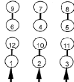
LINE 460 VOLT RUN
