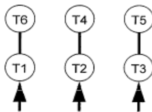
460 VOLT CONNECTION
