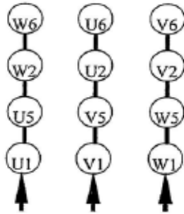
LINE 230 VOLT CONNECTION
