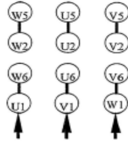
LINE 460 VOLT CONNECTION
